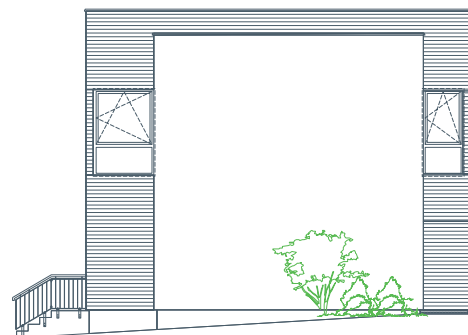
pohľad bočný
