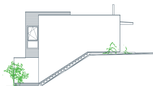
pohľad bočný
